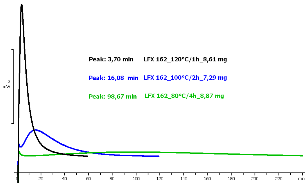
Obr. 2: Závislost rychlosti reakce na čase při konstantních teplotách vytvrzování 80, 100 a 120°C, měřeno na DSC.
