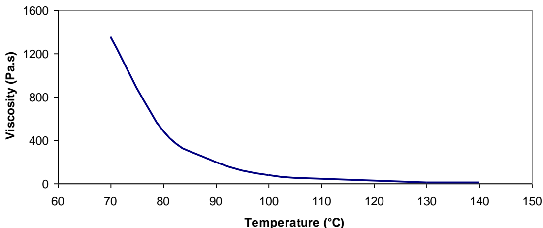
Obr. 3: Závislost viskozity na teplotě
