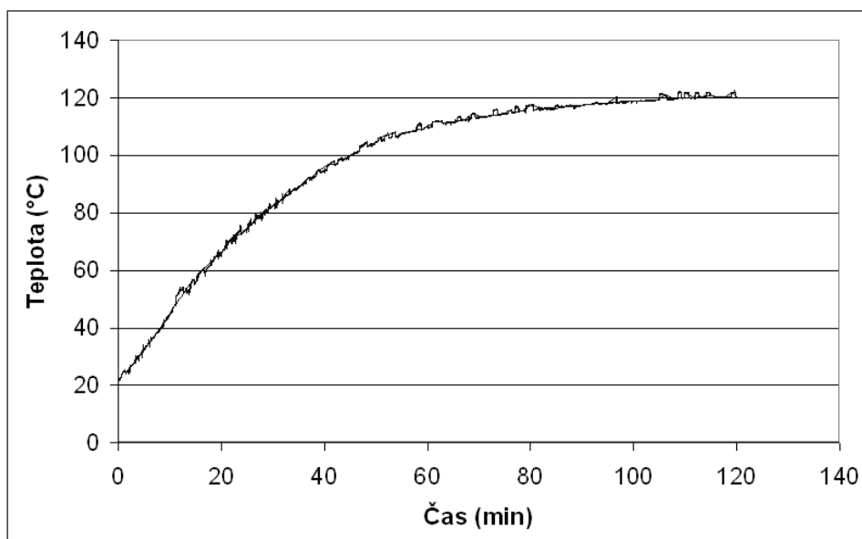
Obr. 4: Závislost teploty uprostřed 2,3mm tlusté kompozice uhlíková tkanina - Letoxit Foil LFX 162 na čase. Vytvrzováno pod vakuem v ocelové formě volně položené v sušárně při 120°C.
