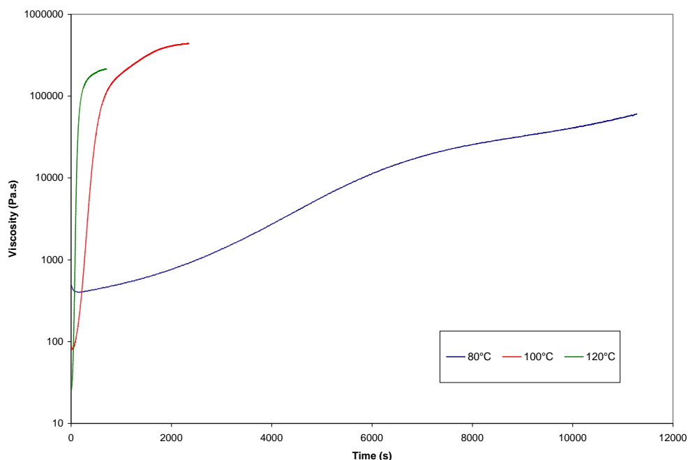
Obr. 1: Závislost viskozity LFX 162 na čase při různých teplotách
